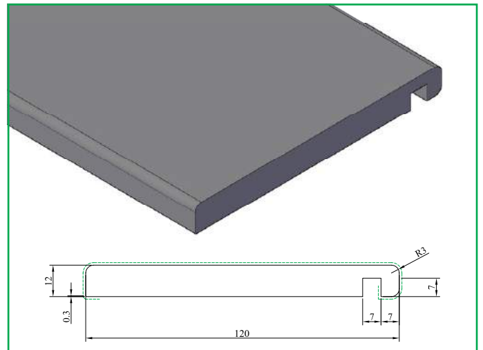
KDK 103 Koplat 12x120 mm
