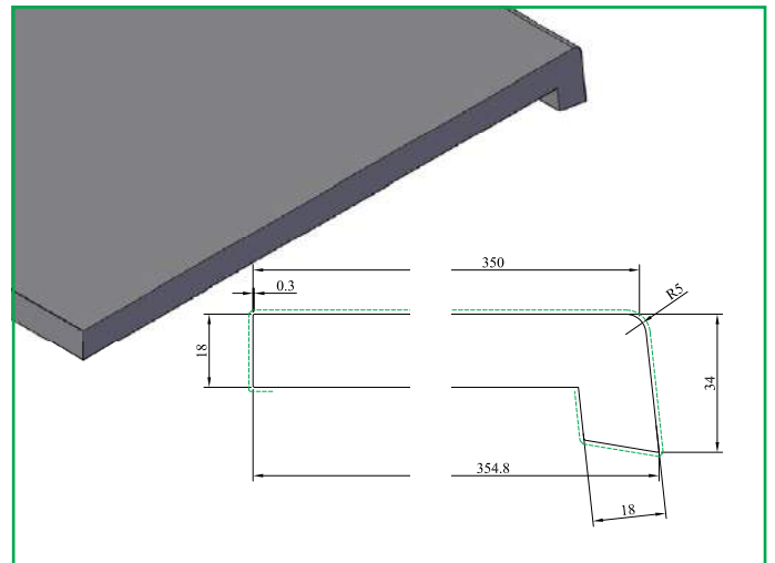
VB 554 SP Vensterbank 350 mm
