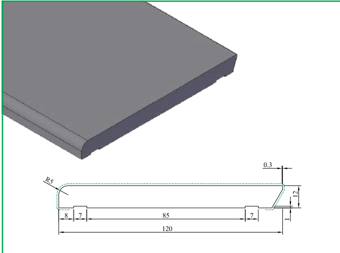
PL 709 Plint 12x120 mm
