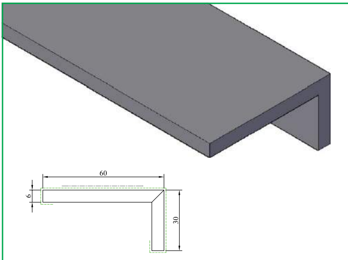
KDH 406 Hoek 6x30x60 mm
