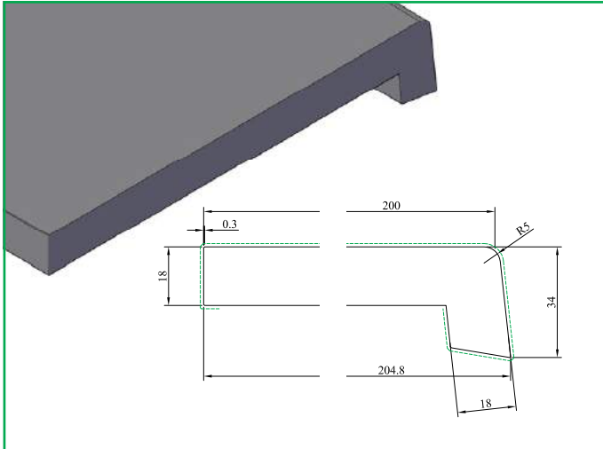
VB 551 SP Vensterbank 200 mm
