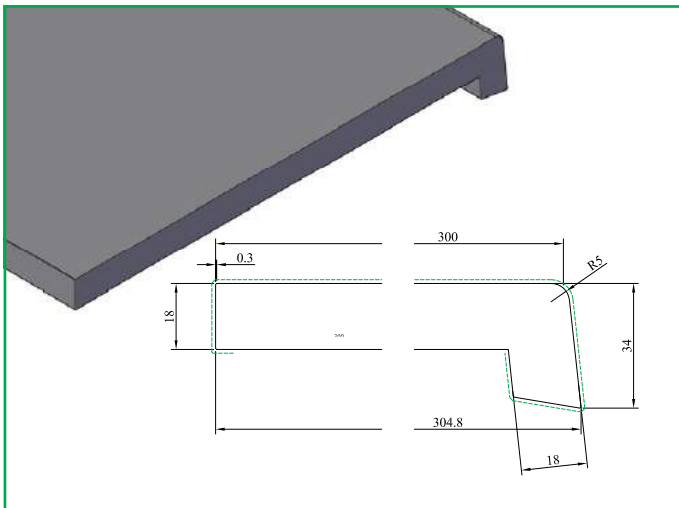
VB 553 SP Vensterbank 300 mm
