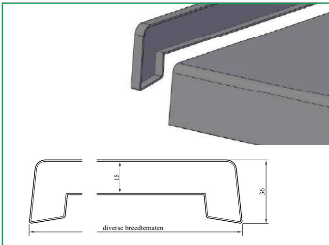
TBH 007 Vensterbank kopafwerking 36x600 mm
