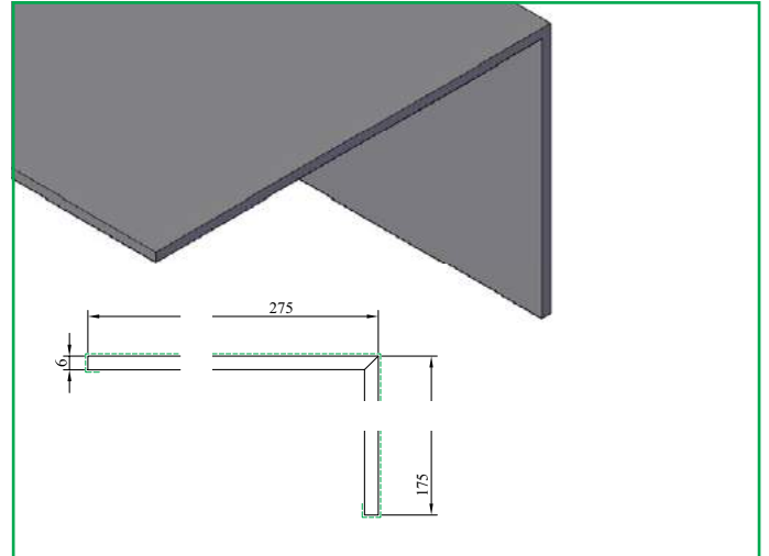
LK 601 Leidingkoker 6x175x275 mm
