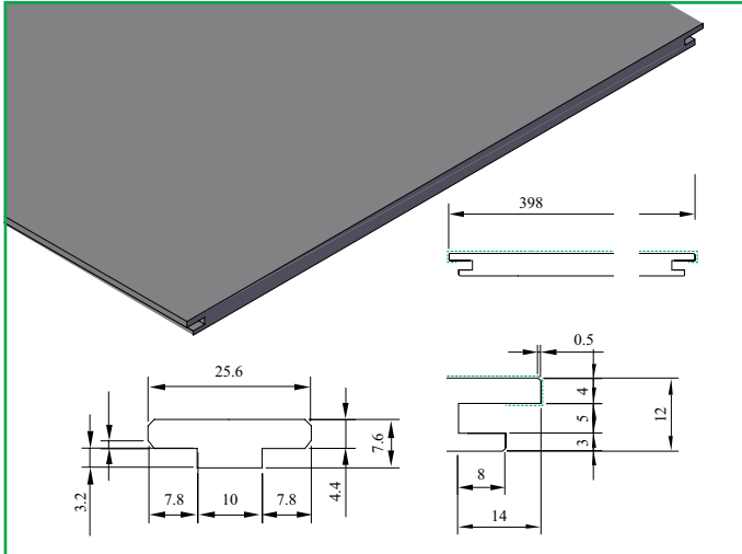
KDP 222 Wand/plafondpaneel 12x398 mm / TBH 016 koppelveer
