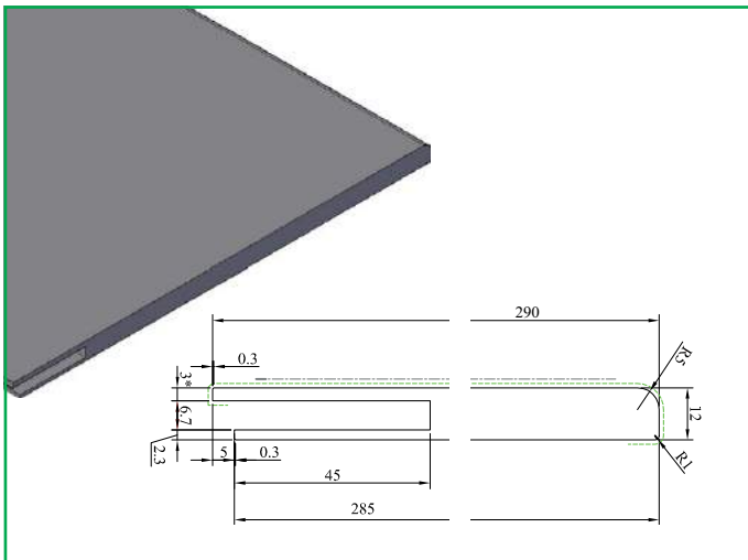
KDP 220 Plaat 12x290 mm
