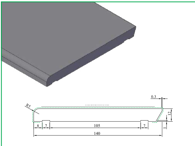
PL 711 Plint 12x140 mm
