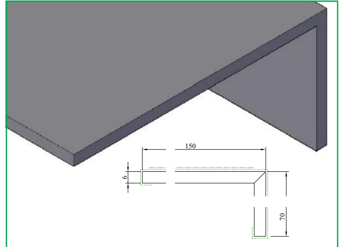
KDH 405 Hoek 6x70x150 mm
