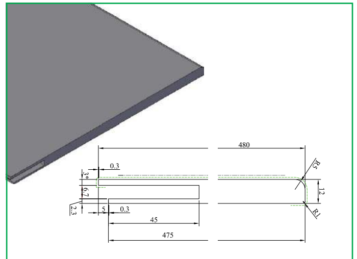
KDP 221 Plaat 12x480 mm
